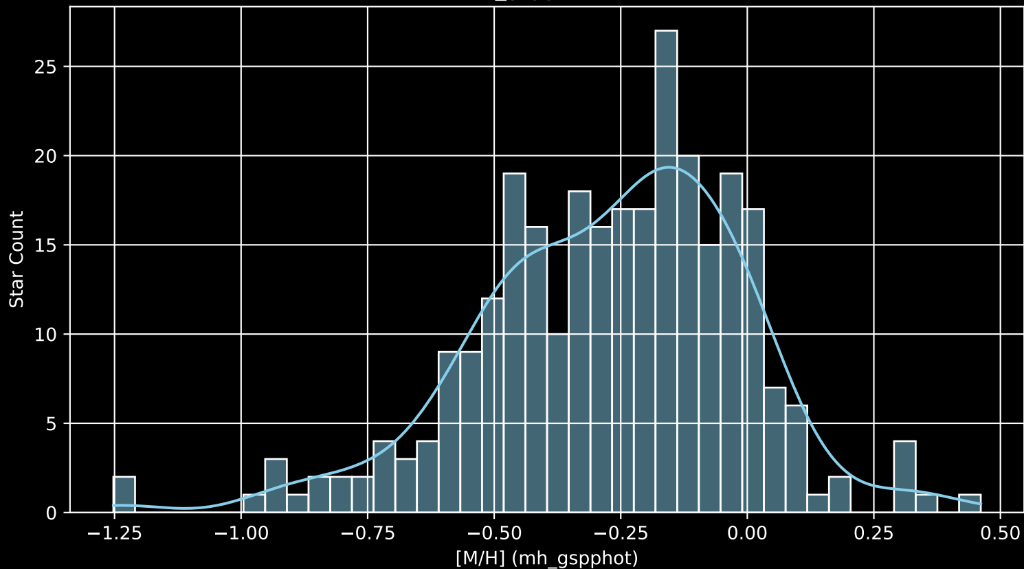
GALAH DR4 Field: [9404] [M/H] (mh_gspphot) (n= 287)
