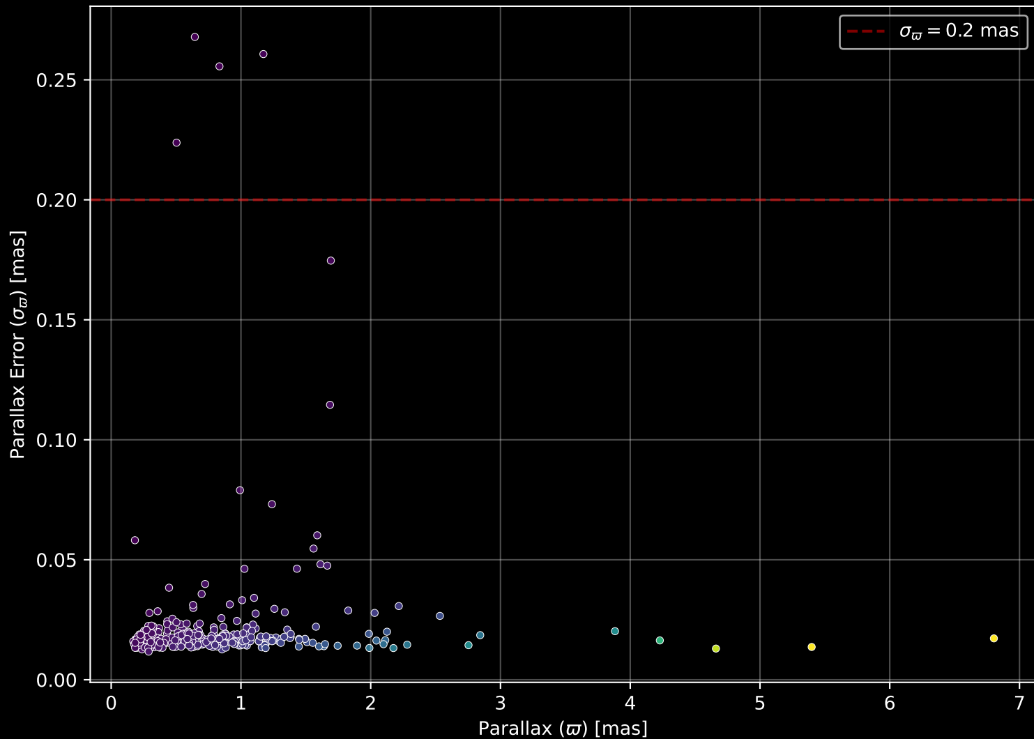
GALAH DR4 Field: [9404] Parallax Quality (n= 289)
