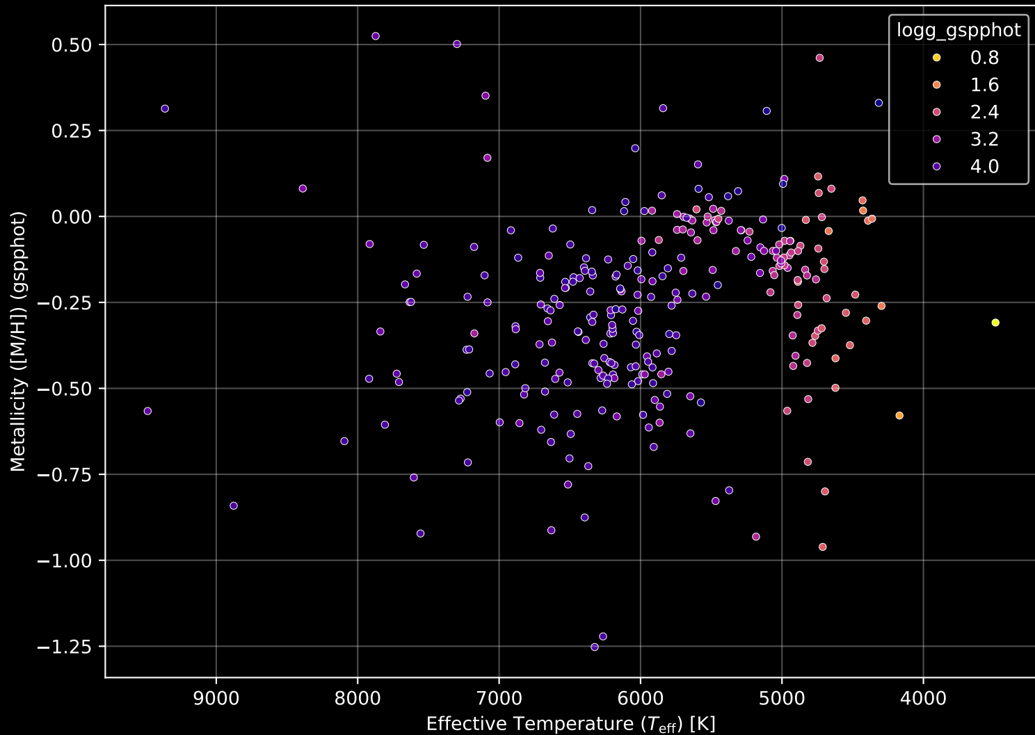
GALAH DR4 Field: [9404] Stellar Population Parameters (n= 289)
