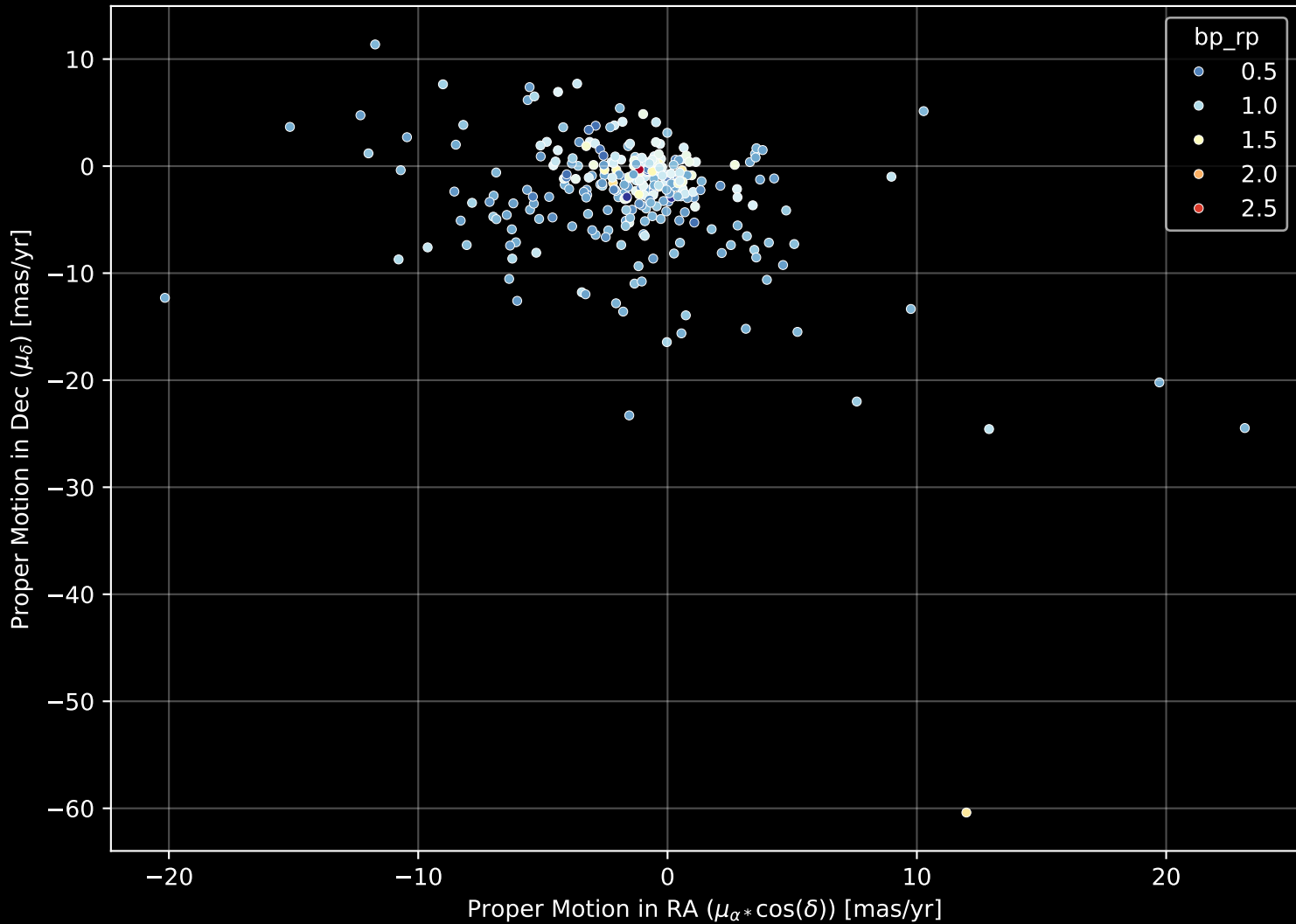
GALAH DR4 Field: [9404] Proper Motion Diagram (n= 289)
