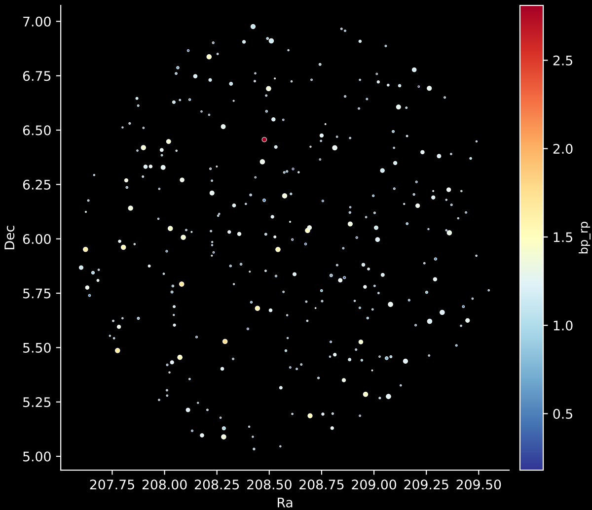
GALAH DR4 Field: [9404] Stars: 289
